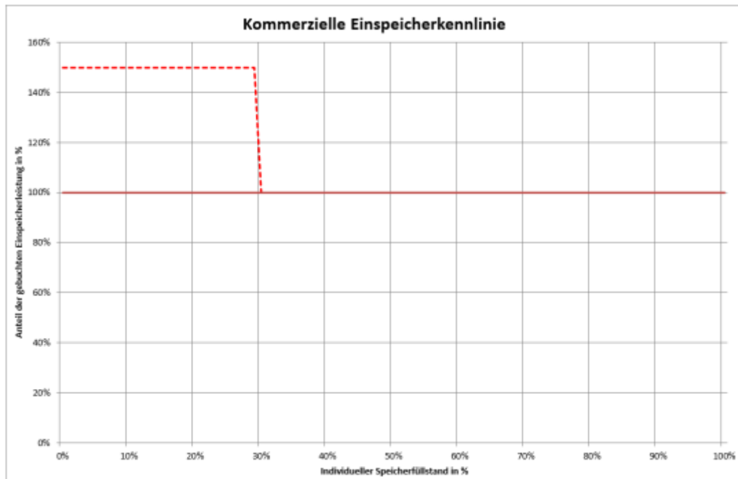
Abbildung 2: Kommerzielle Einspeicherkennlinie des Speichers Frankenthal
