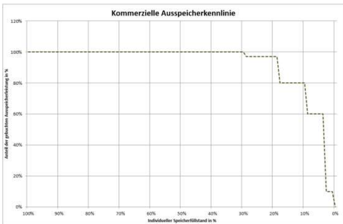
Abbildung 1: Kommerzielle Ausspeicherkennlinie des Speichers Frankenthal
