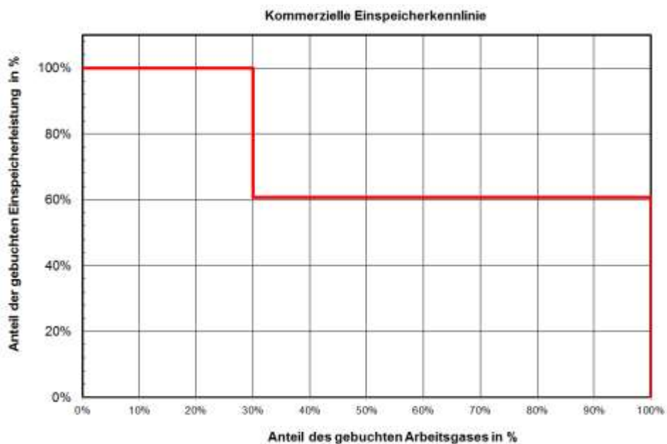
Abbildung 2: Kommerzielle Gesamt-Einspeichererkennlinie des Speichers Frankenthal
