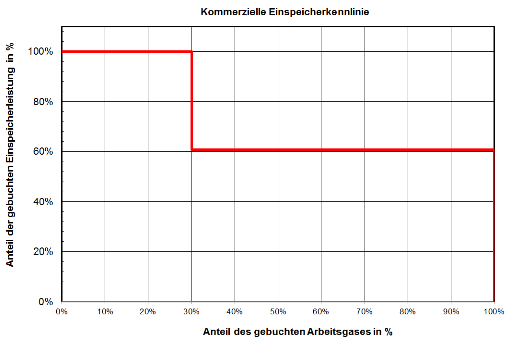
Abbildung 2: Kommerzielle Gesamt-Einspeicherkennlinie des Speichers Frankenthal
