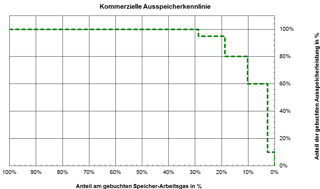
Abbildung 1: Kommerzielle Gesamt-Ausspeicherkennlinie des Speichers Frankenthal
