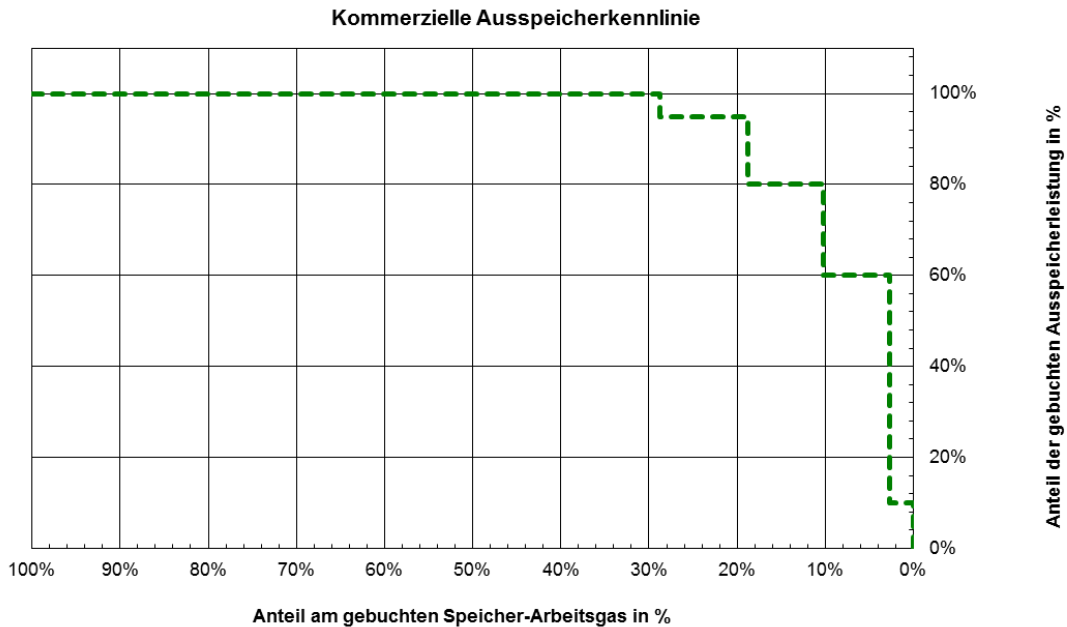
Abbildung 1: Kommerzielle Gesamt-Ausspeicherkenlinie des Speichers Frankenthal
