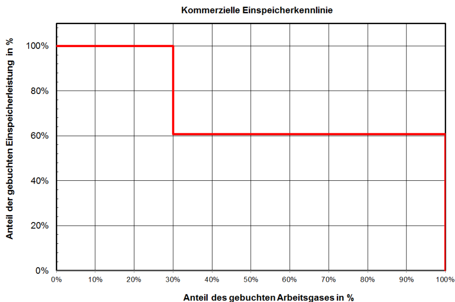
Abbildung 2: Kommerzielle Gesamt-Einspeicherkenlinie des Speichers Frankenthal
